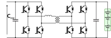
(d) Dual Active Bridge dc-dc Converter Interface
