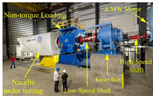
5-MW dynamometer
